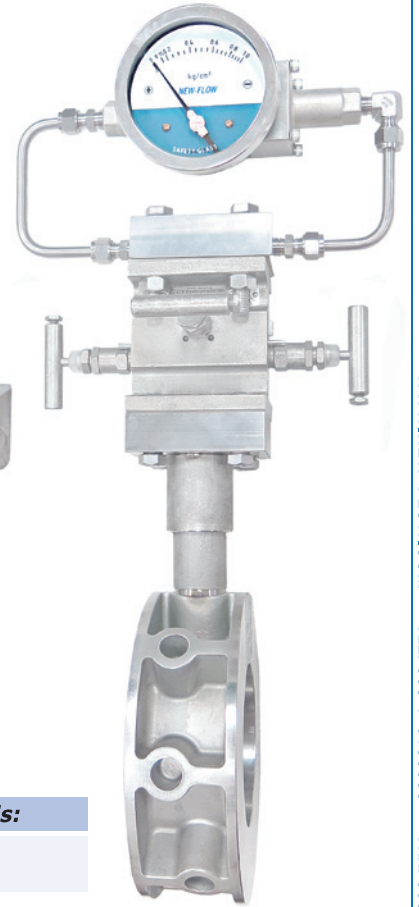
D/P Gauge
